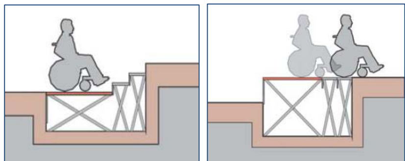
Figura 29 e Figura 30- Esempio di piattaforma elevatrice e scomparsa
