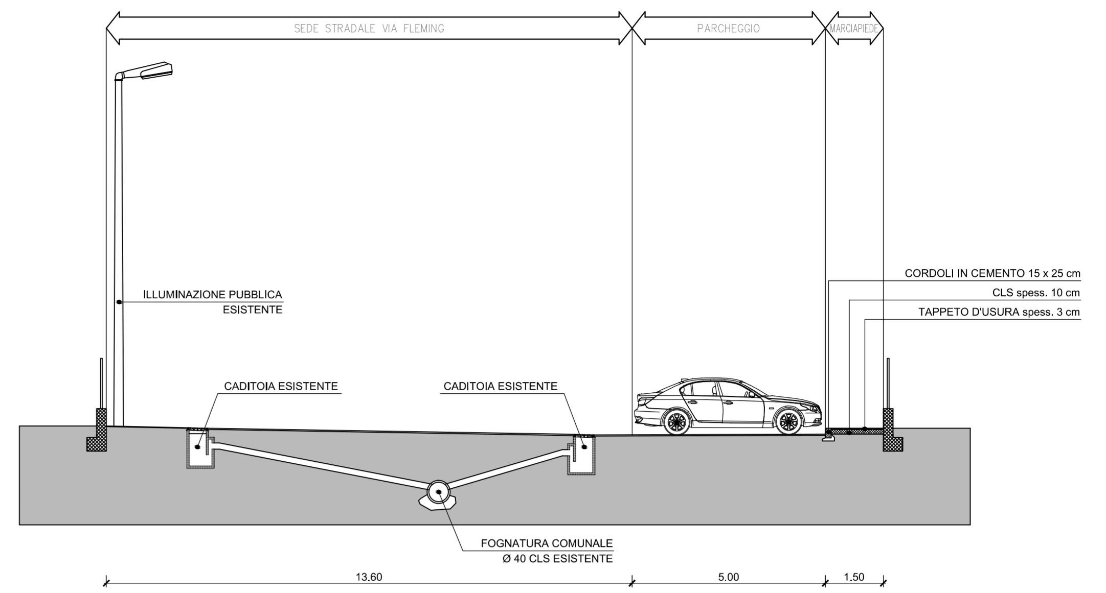
SEZIONE A-A
