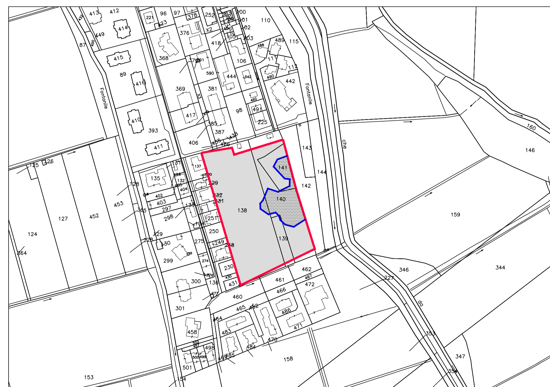
ESTRATTO MAPPA AREA BOSCATI Foglio 13 - Mappali 138 parte - 139 parte - 140 parte - 141 parte Scala 1:2000
